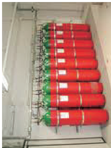
Impianto a gas inerti (es.: argon IG-02)
